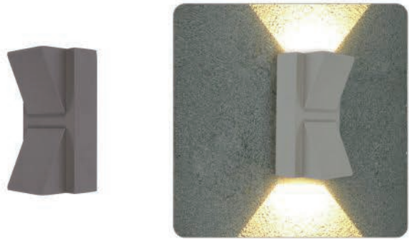
Model 型号 : DFB-8006 Power 功率 : 6W Size 尺寸 : 142x60x40mm Colour Temperature 色温 : 2700K/3000K/4000K/6000K Input Voltage 输入电压 : AC85-265V 50-60Hz Product Colour 灯体颜色 : Black/Grey/White 砂黑 / 砂灰 / 砂白 Material 主要材质 : Die-casting aluminum/Glass 压铸铝 / 玻璃
